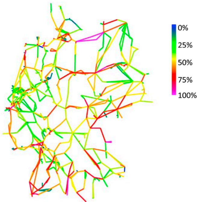
ABBILDUNG 36: AUSLASTUNG DES ERWEITERTEN SZENARIO B 2033 IM GRUNDFALL
