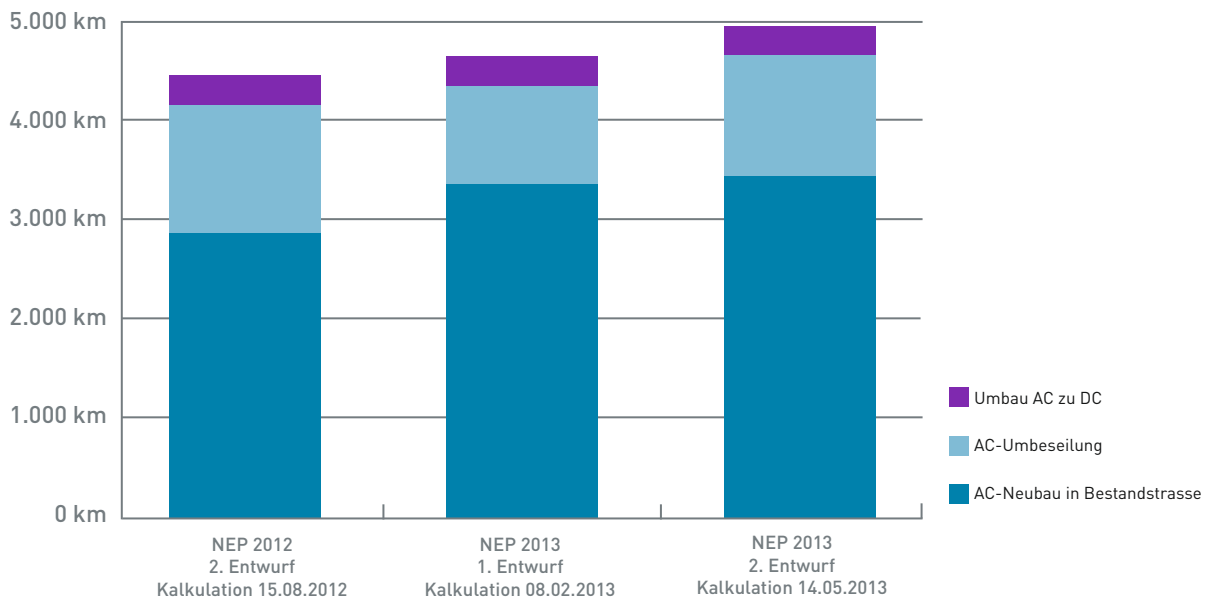
ABBILDUNG 45: TRASSENVERSTÄRKUNGEN IM BESTAND
