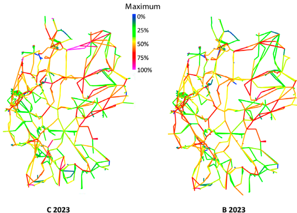
ABBILDUNG 37: GEGENÜBERSTELLUNG DER NETZAUSLASTUNG DER SZENARIEN C 2023 UND B 2023 IM GRUNDFALL BEI GLEICHER NETZTOPOLOGIE
