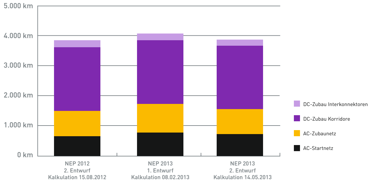
ABBILDUNG 46: NEUBAUTRASSEN
