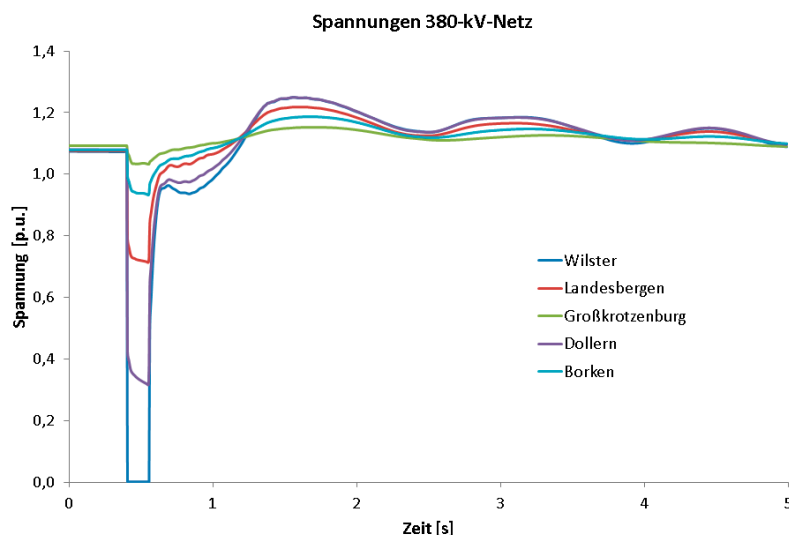
ABBILDUNG 43: 3-POLIGER KURZSCHLUSS IN DER NÄHE DES UW WILSTER, AUSFALL EINES STROMKREISES NACH DOLLERN (FEHLERDAUER: 150 MS)
