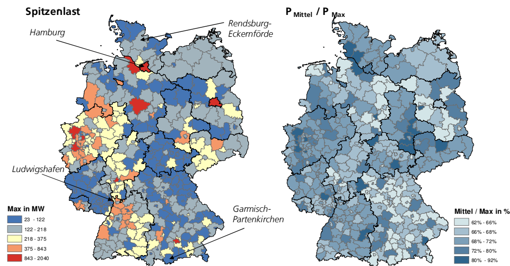
Abbildung 42: Spitzlast (links) und Lastfaktor P_{Mittel} / P_{Max} (rechts) auf Landkreisebene im Basisjahr
