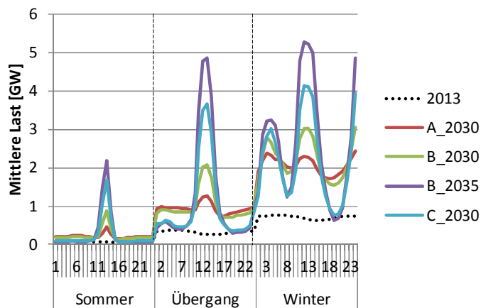
Abbildung 38: Mittlerer Lastverlauf der Wärmepumpen für Werkzeuge in Sommer, Übergangszeit und Winter im Basisjahr und für das Jahr 2030 bzw. 2035
