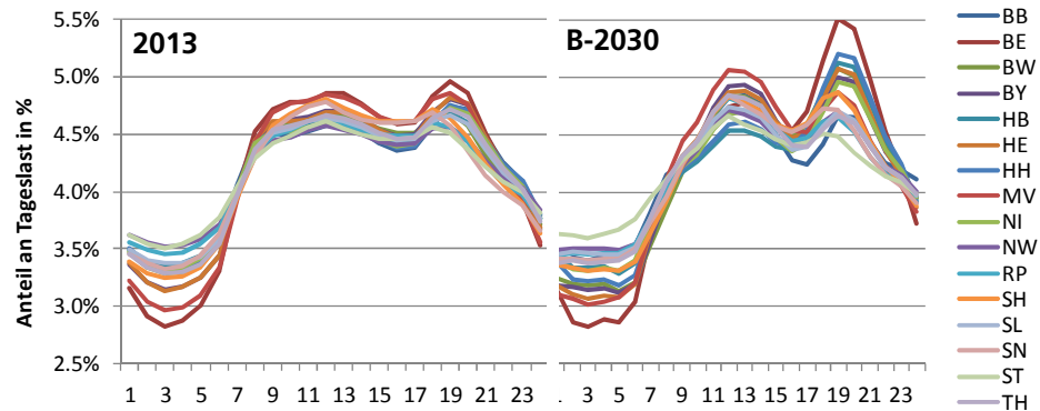
Abbildung 49: Verteilung der Last über den Tag im Basisjahr und im Szenario B in 2030 für die Bundesländer an einem mittleren Winter-Werktag
