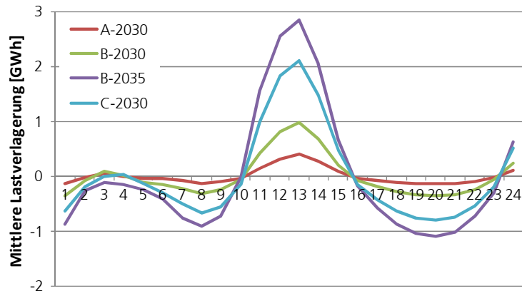
Abbildung 40: Mittlere Lastverlagerung – Summe über alle lastmanagementfähigen Anwendungen
