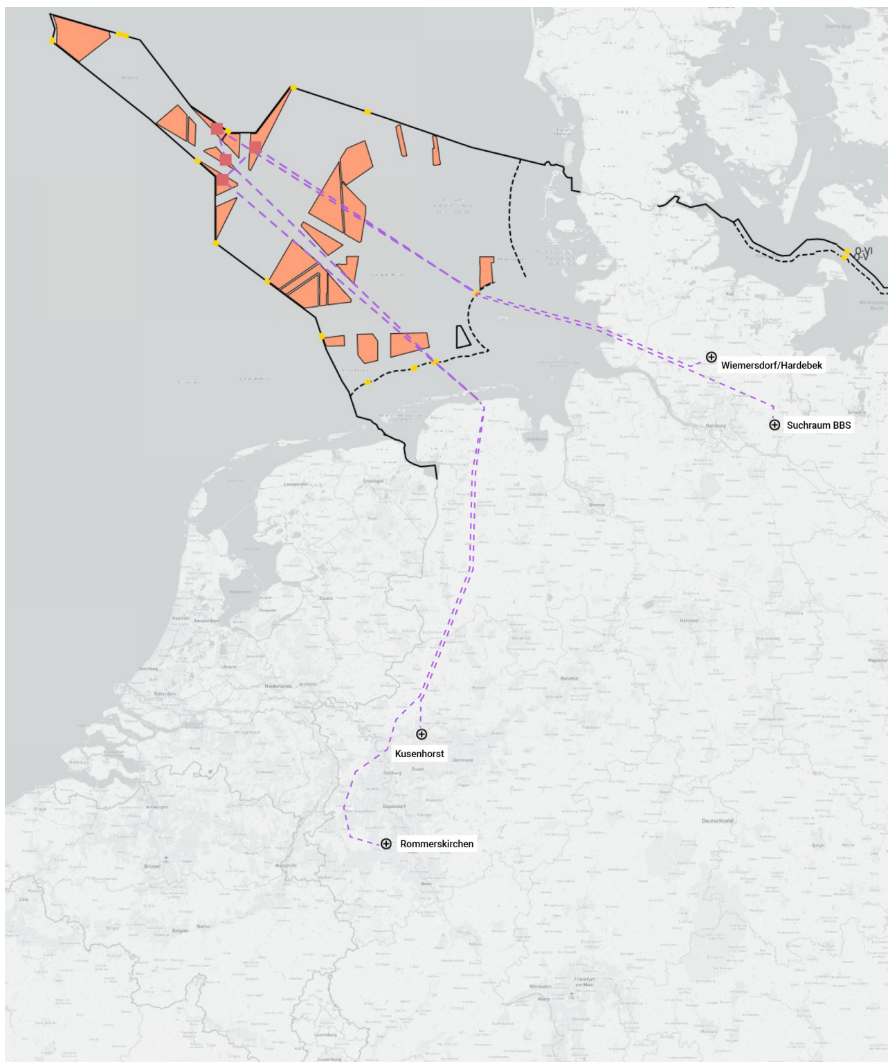
Abbildung 58: Nationale Offshore-Vernetzung
