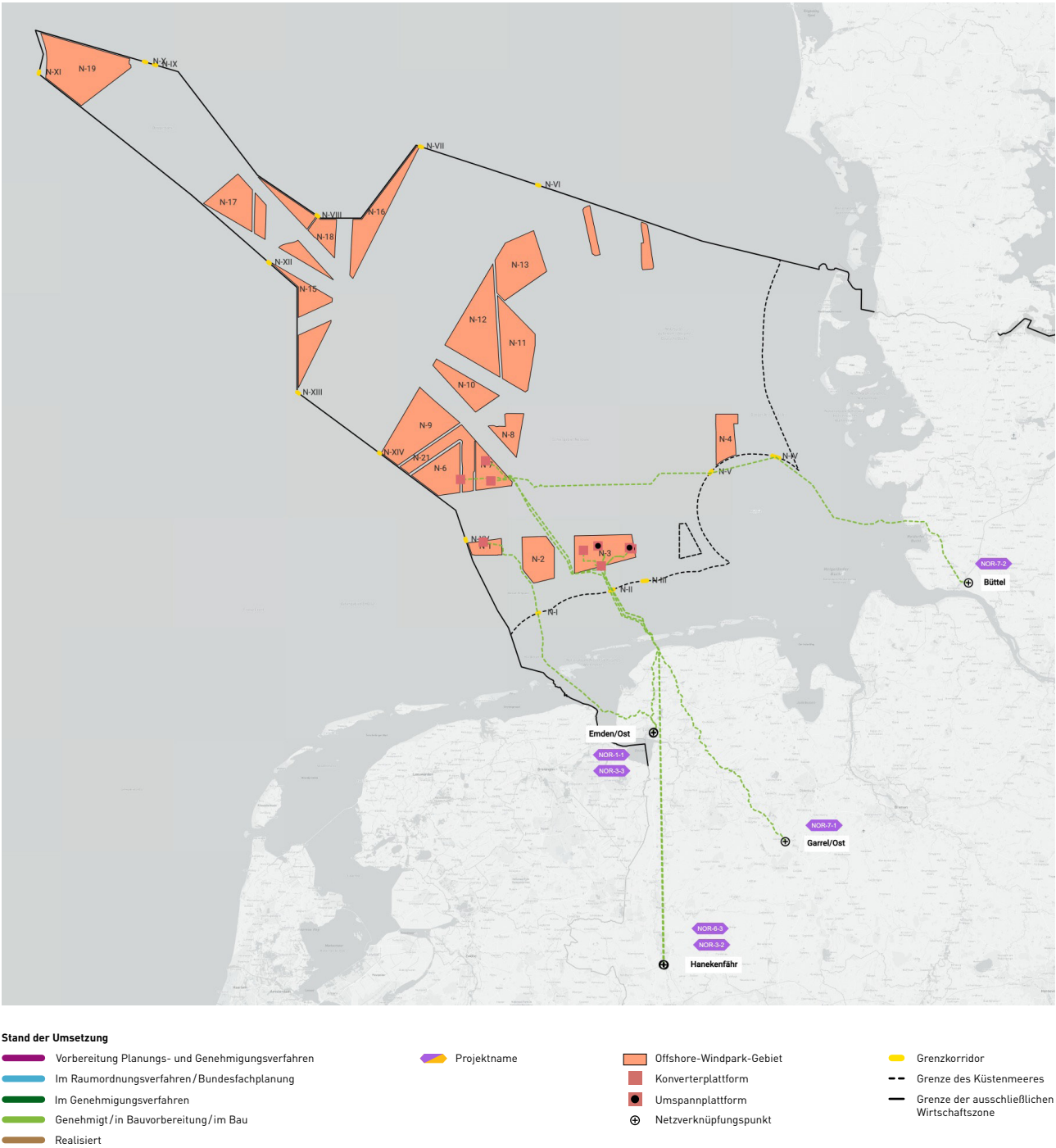
Abbildung 49: Offshore-Startnetz Nordsee
