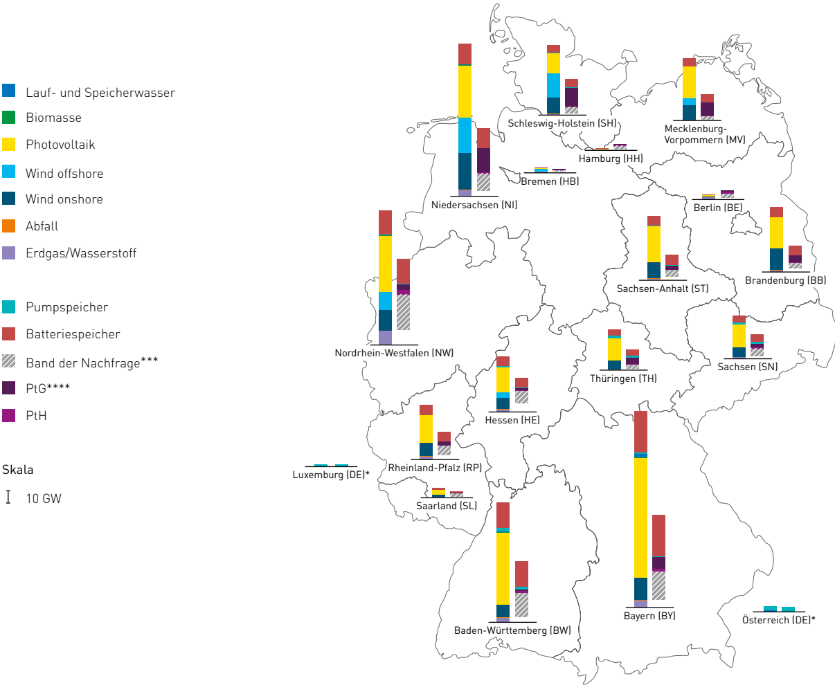
Abbildung 17: Installierte Leistungen je Bundesland im Szenario A 2045
